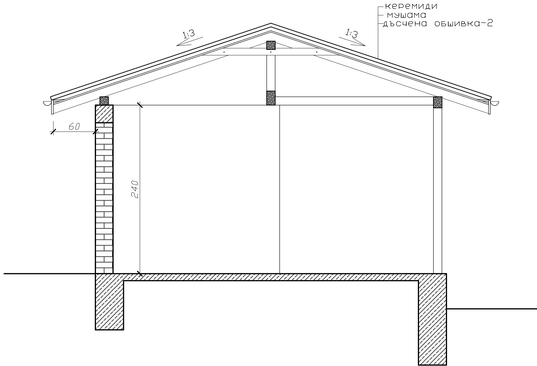
НАПРЕЧЕН РАЗРЕЗ
